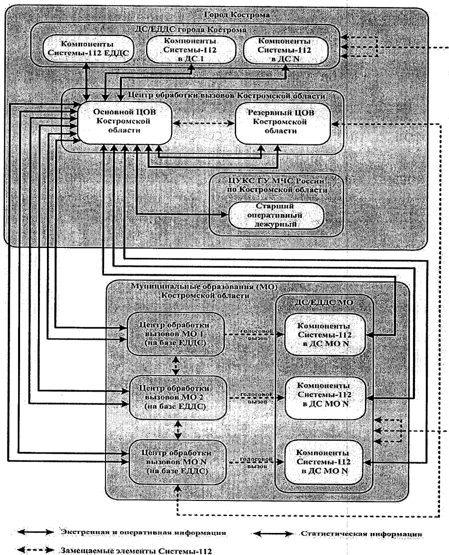
Рисунок. Схема построения системы-112 Костромской области
